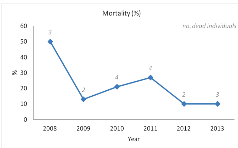
Fig. 19. Evolution du taux de mortalité (Auteurs: Aleix Millet / Mario Álvarez).
