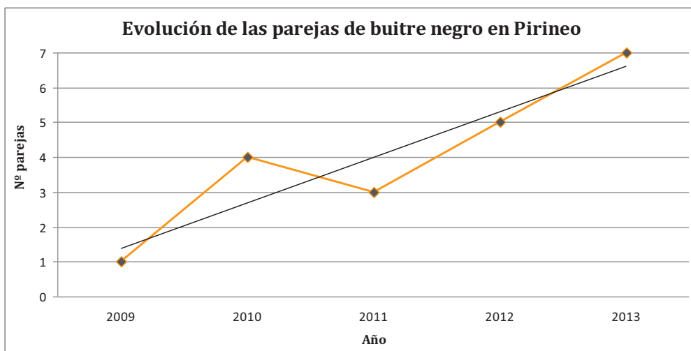
Fig. 5. Évolution des couples de vautours moines dans les Pyrénées. N° de couples (Auteurs : Aleix Millet / Mario Álvarez).
